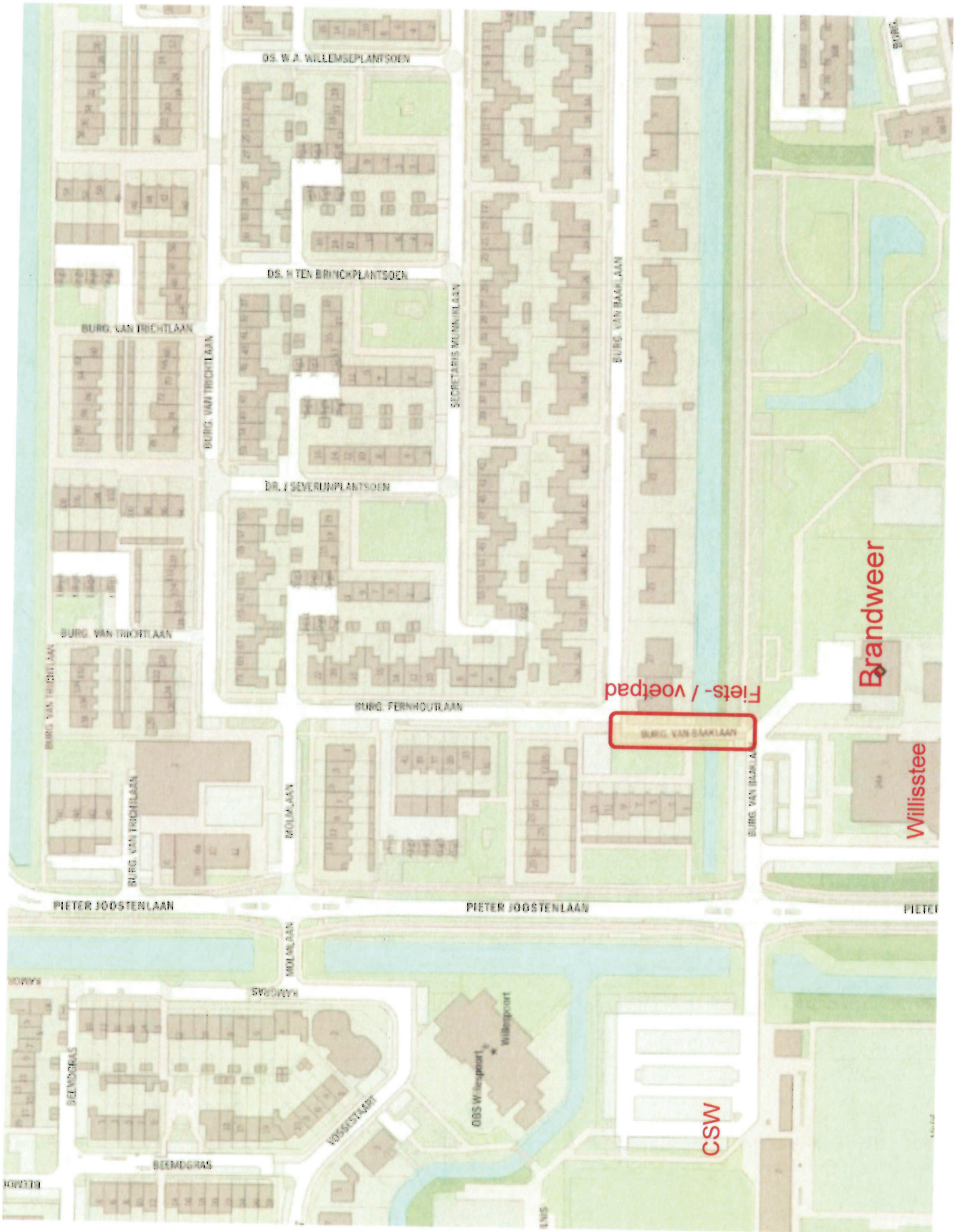
Situatietekening - Fiets- / voetpad
